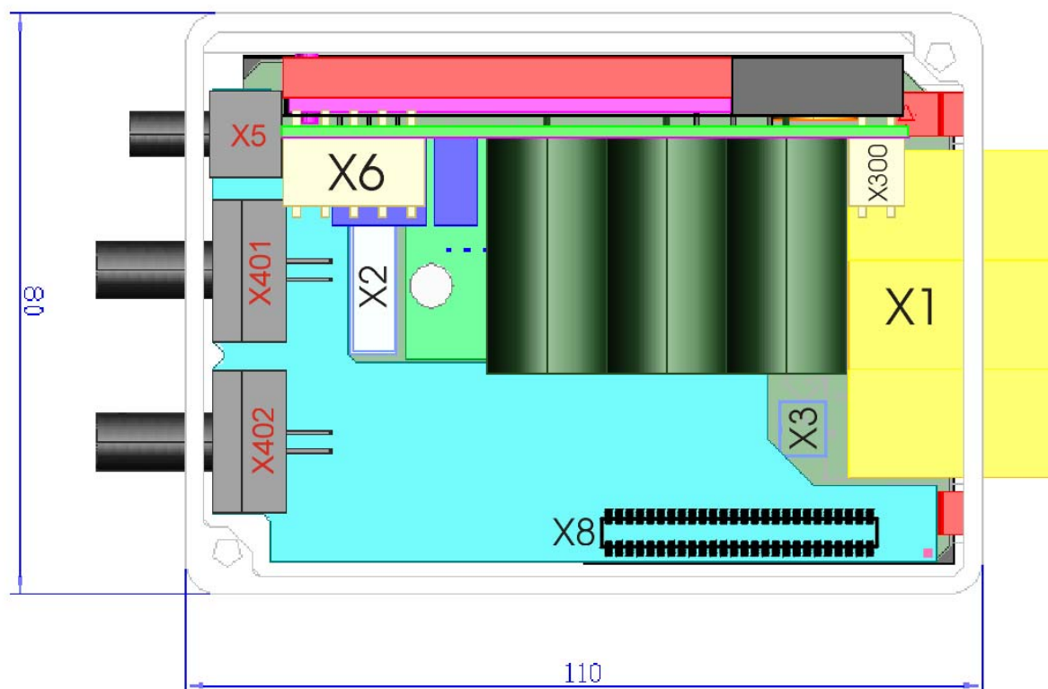
Abbildung 5: Anordnung Steckverbinder MDRM 230/2-6 FB – Draufsicht des Gerätes
