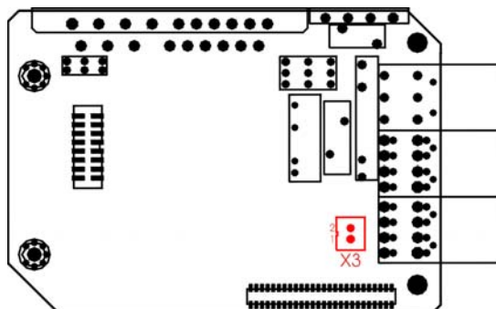
Abbildung 13: Anschluss Haltebremse
