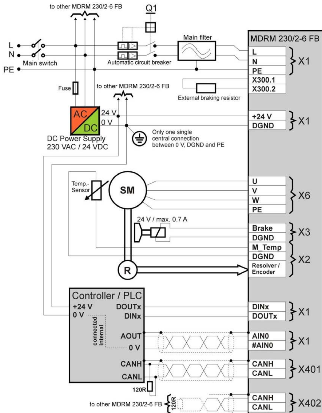
Abbildung 9: Anschluss an Spannungsversorgung, Steuerung und Motor
