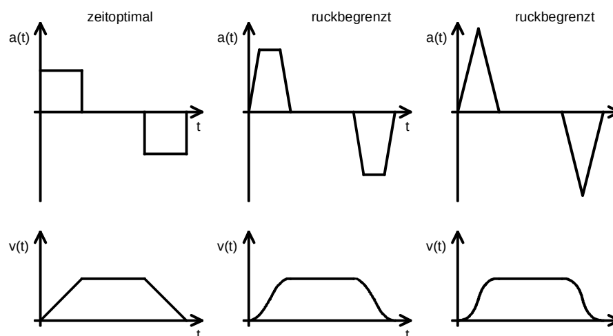
Abbildung 3: Fahrprofile des Servopositionierreglers MDRM 230/2-6 FB
