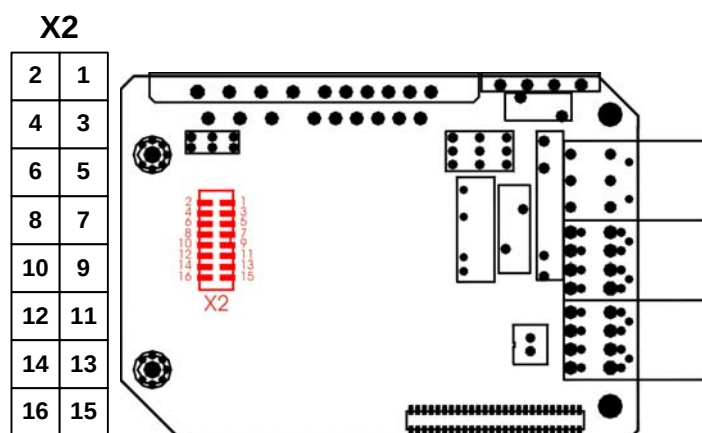
Abbildung 12: Anschluss Winkelgeber
