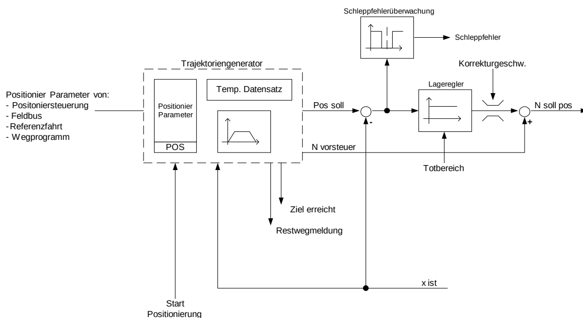
Abbildung 2: Blocksaltbild Positioniersteuerung
