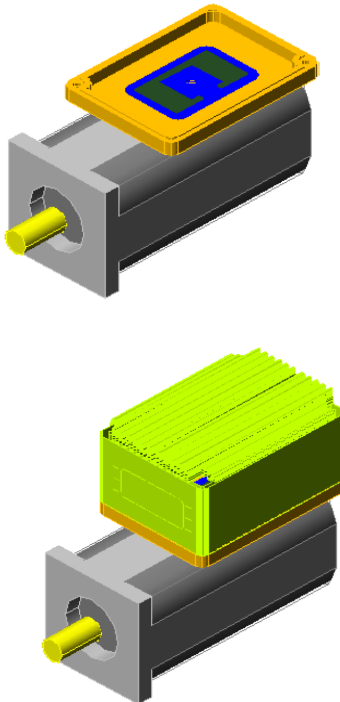
Abbildung 7: MDRM 230/2-6 FB Montagebeispiel – Synchron Servo Motor, Montageplatte mit Bremswiderstand und Servopositionierregler MDRM 230/2-6 FB
